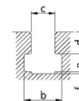
T-SLOT
