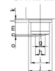
SPINDLE
